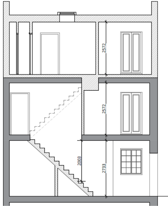
Section A-A Scale: 1:50 @ A2
