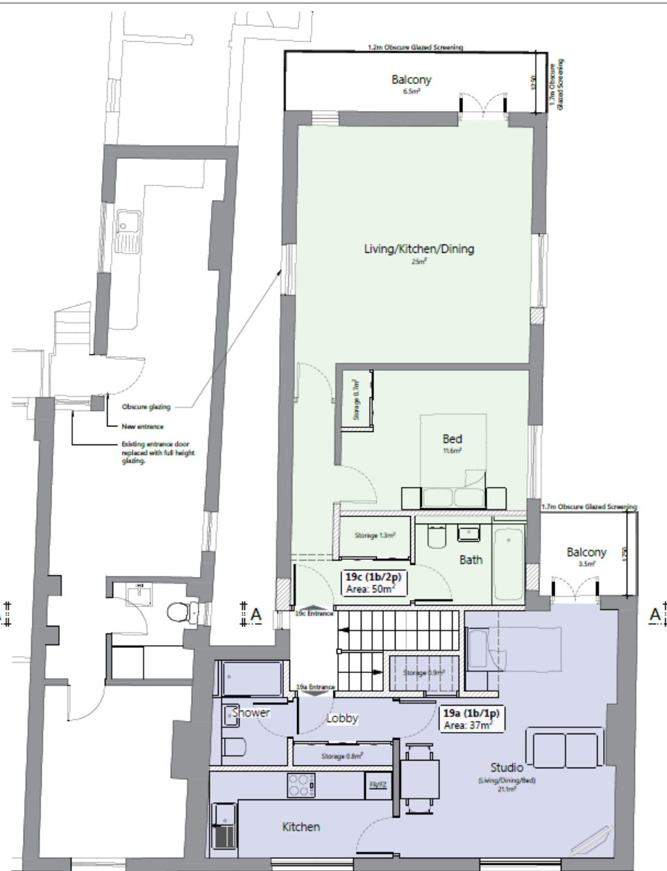
First Floor Scale: 1:50 @ A2
